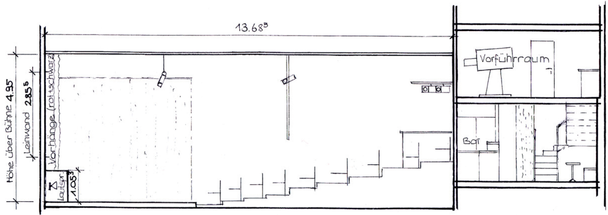
Schnitt A-A
